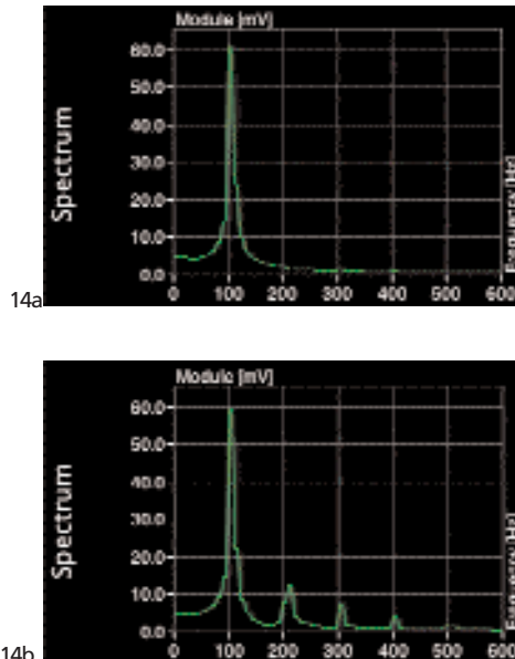
14 Modulationsspektren von Glühlampe (14a) und Kompaktleuchtstofflampe (14b).
