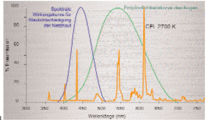
2 Spektrum einer Kompaktleuchtstofflampe mit der Bezeichnung »Nature Color« mit einer Farbtemperatur von 6500 K und einem angeblichen Farbwiedergabeindex von RA (92), laut Herstellerangaben auch für »Therapeutische Anwendungen« geeignet, allerdings ohne therapeutische CE-Kennzeichnung.
