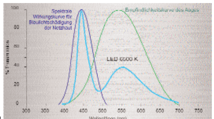
4 Spektrum einer Weißlicht-LED mit starker Betonung im kurzwelligen Bereich.
