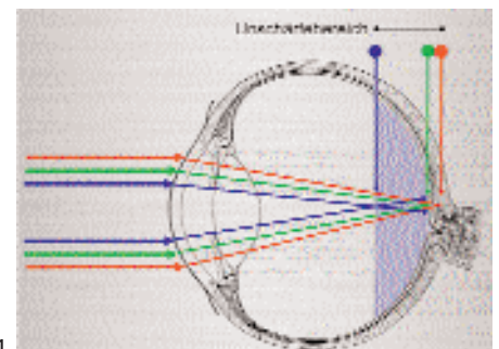
11 Abb. 11: Die chromatische Aberration im Auge führt zu verschiedenen Schärferebenen für die unterschiedlichen Wellenlängen des Lichts.
